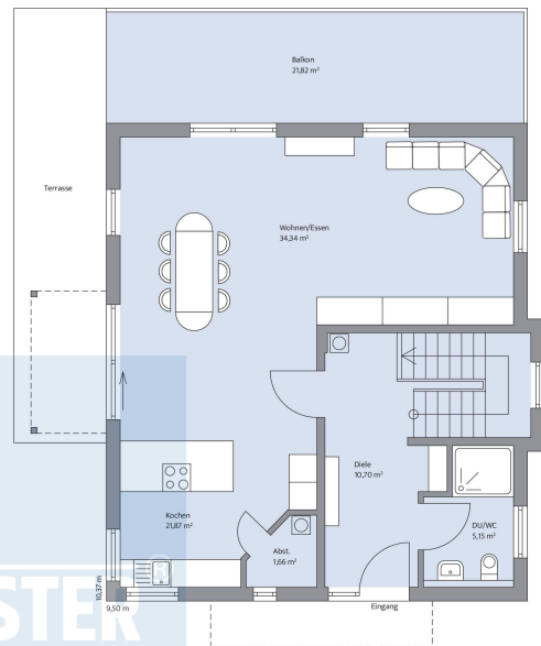
Haus Echterkamp Grundriss
