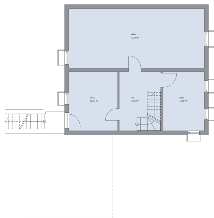
Haus Falkenberg Grundriss KG
