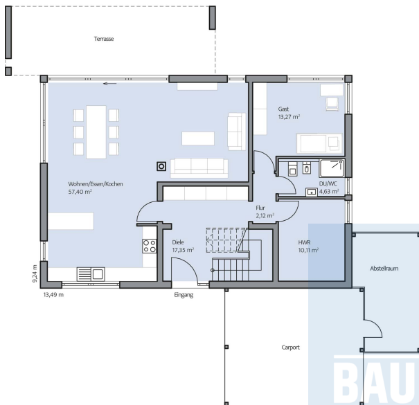
Haus Zoellner Grundriss
